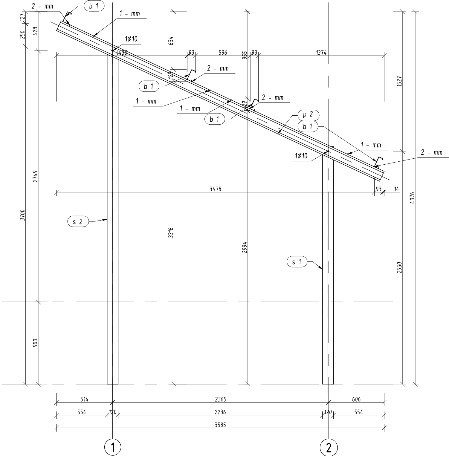
Widok z boku skala 1:20
